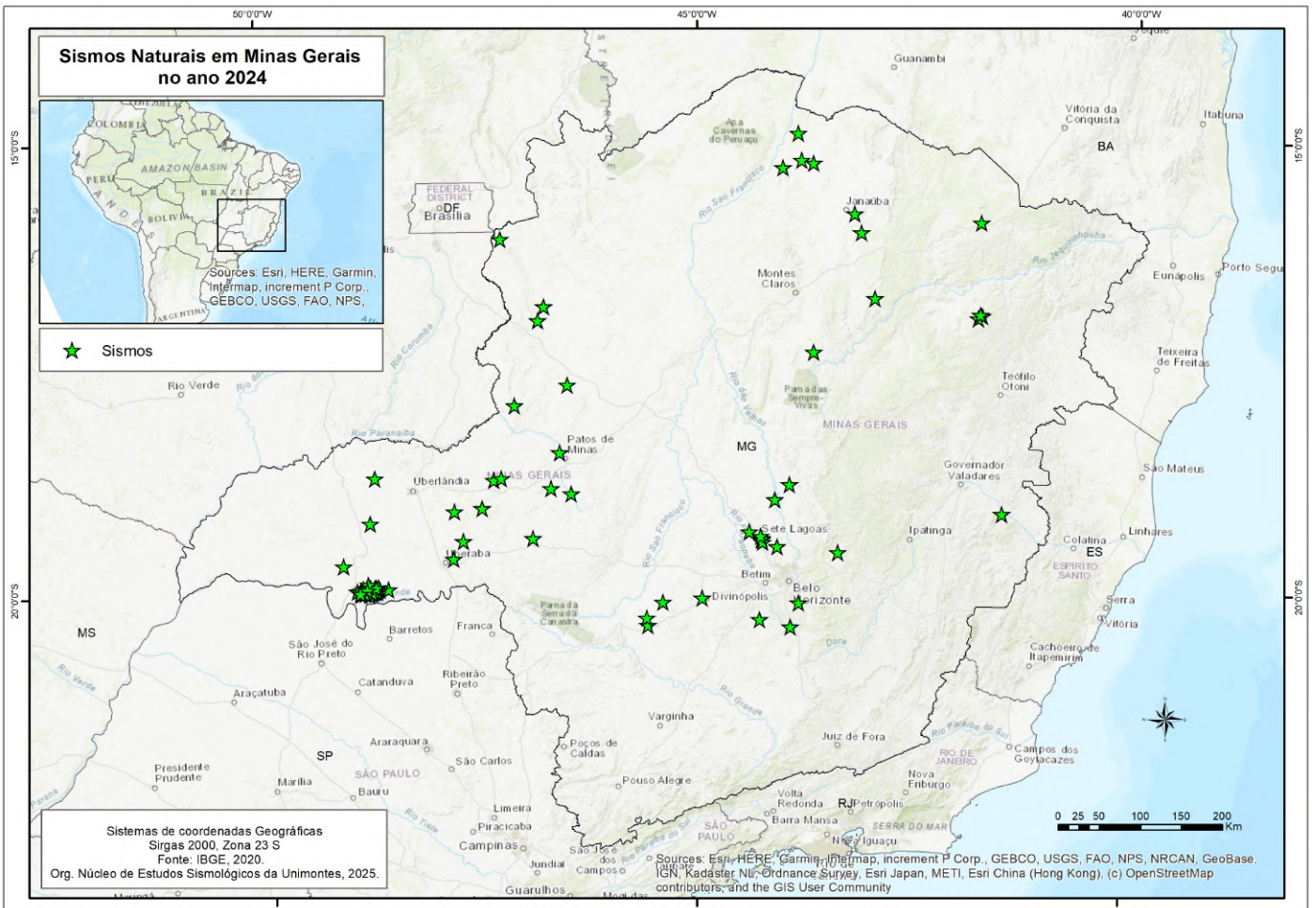
Mapas 1 e 2: Sismos naturais ocorridos em Minas Gerais em 2024
