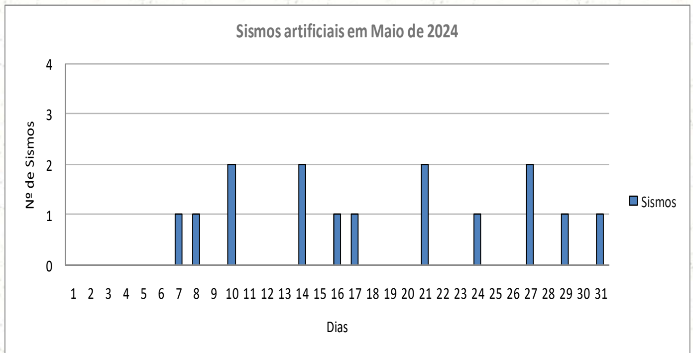
Gráfico 2: Sismos artificiais (detonações em pedreiras) ocorridos em Montes Claros em Maio de 2024
