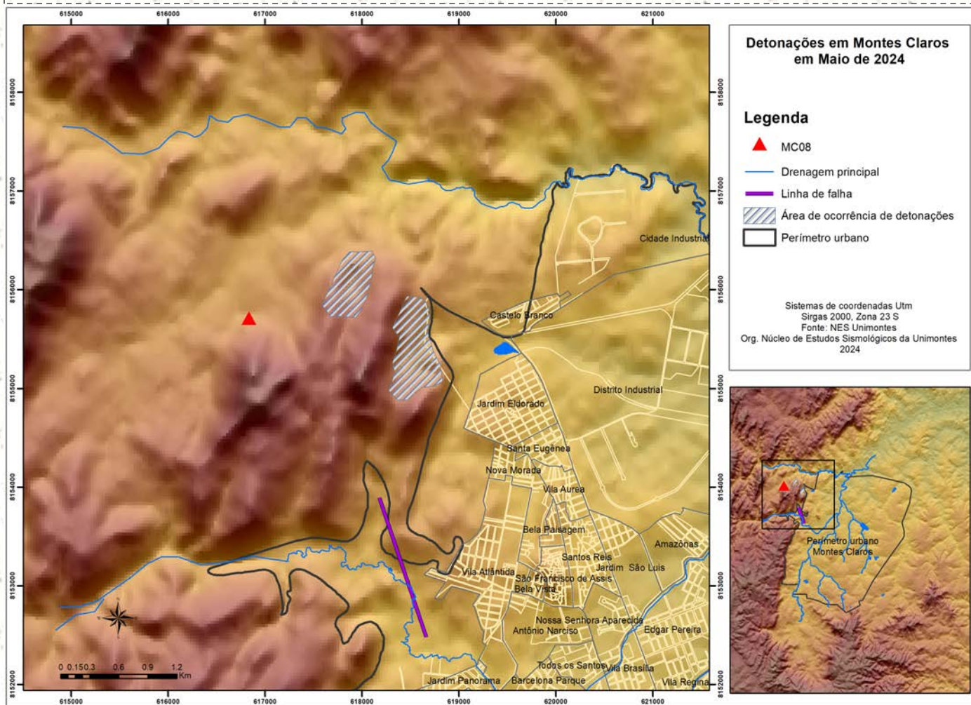
Mapa 02 : Sismos artificiais (detonações em pedreiras) em Montes Claros em Maio de 2024.
