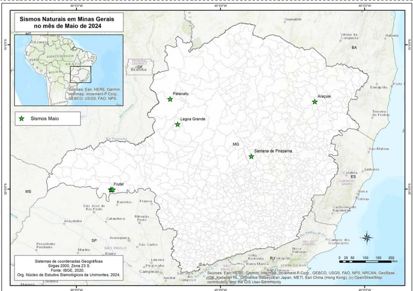
Mapa 1: Sismos naturais ocorridos em Minas Gerais em Maio de 2024
