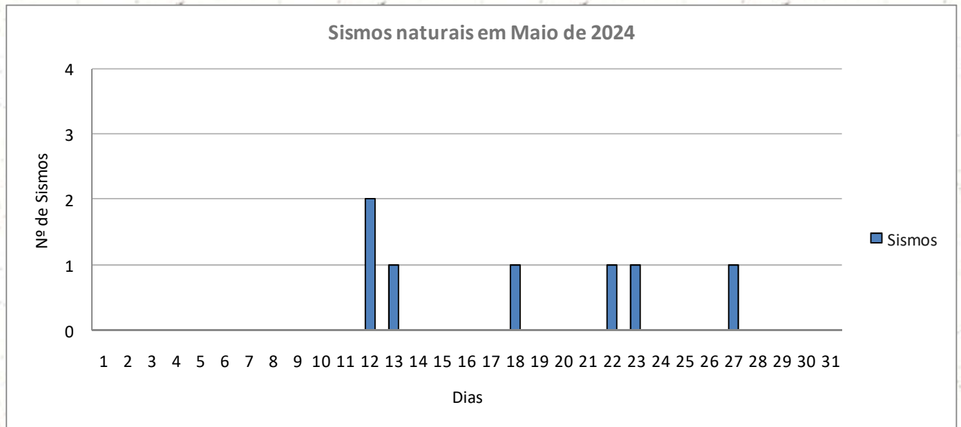
Gráfico 1 : Sismos naturais ocorridos em Minas Gerais em Maio de 2024
