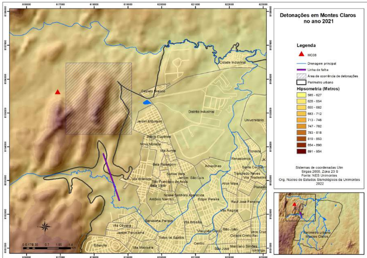
Mapa 02 : Sismos artificiais (detonações em pedreiras) em Montes Claros no ano 2021
