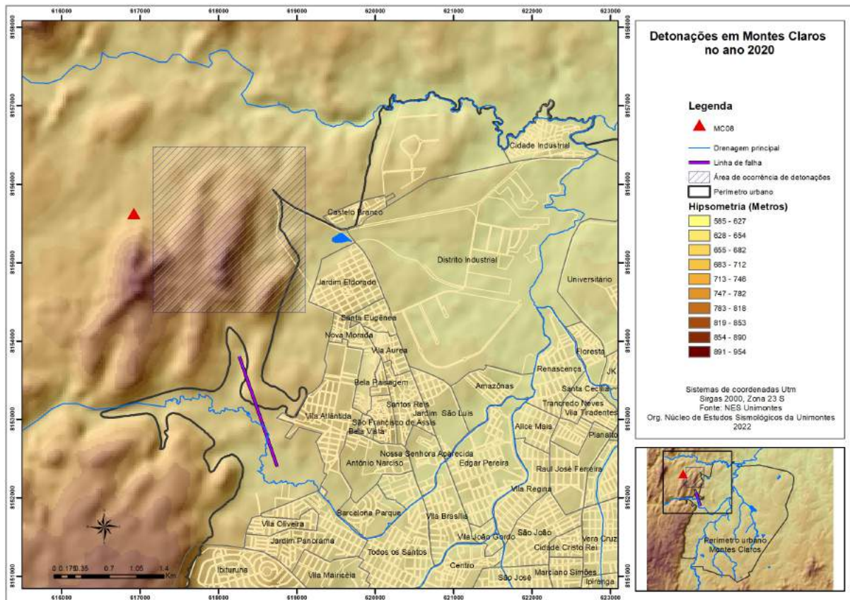
Mapa 02 : Sismos artificiais (detonações em pedreiras) em Montes Claros no ano 2020
